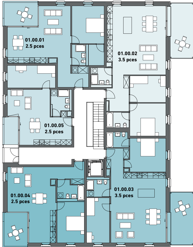
Rez-de-chaussée
